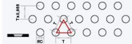
RI / T (nerpressade hål, triangelindelning)
