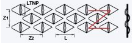
POLR (läpperforering – stängd)
