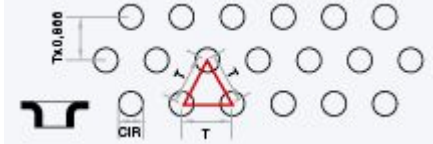
RI / M (nerpressade hål, diagonaldelning)
