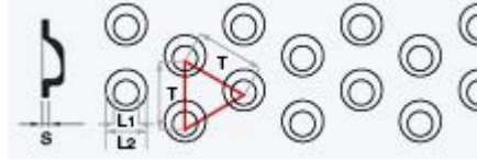
LT / Z (sträckmetall, förskjuten delning)
