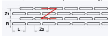
LR / Z (slitshål, förskjuten delning)
