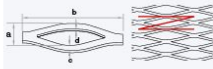
PCLR (läpperforering – öppen)
