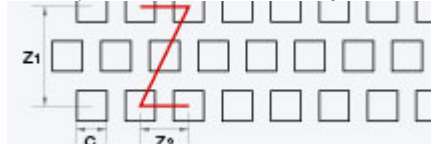
CPRR / M (klöver + hål, diagonaldelning)
