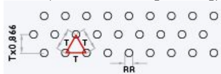
TTR / U (triangulära hål, rektangelindelning)
