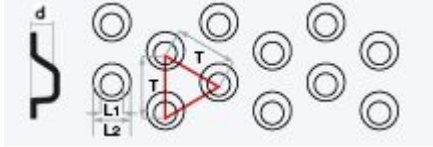
LTNP / Z (ögonlock, förskjuten delning)
