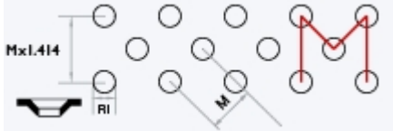
RI / U (nerpressade hål, kvadratdelning)
