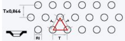
RI / Z (nerpressade hål, förskjuten delning)
