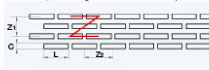
LRDD / U (slitshål, fiskbensdelning)
