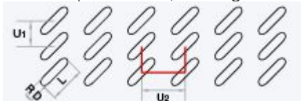
LRD / U (slitshål 45°, rektangeldelning)
