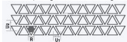
TTR / U (triangulära hål, rektangelindelning)
