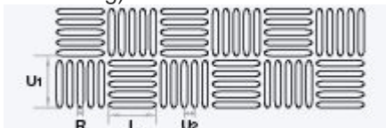
LRD / U (Langlochung diagonal, geradreihig)
