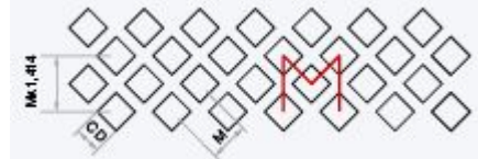
C / Z (Quadratlochung, versetzt)
