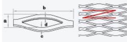
PCLR (Klappenlochung offen)
