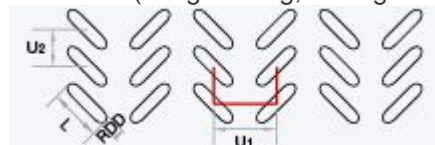
LRDD / U (Langlochung, Fischgrätenanordnung)
