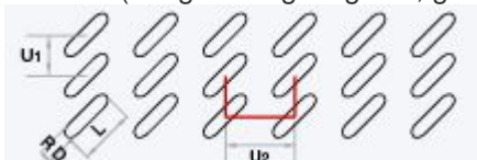
LR / U (Langlochung, geradreihig)
