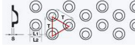
LT / Z (Streckmetall)
