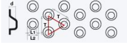
LTNP / Z (Nasenblech, versetzt)
