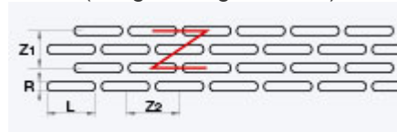
LR / Z (Langlochung, versetzt)
